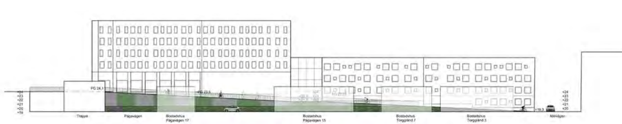
Figur 5. Sektion A-A. Det norra centrumkvarteret som tydligt visar hur kvarteret sluttar 4 meter i höjd, Arkitektlaget och Tyréns. Figuren redovisar ett av många möjliga utbyggnadsalternativ.
