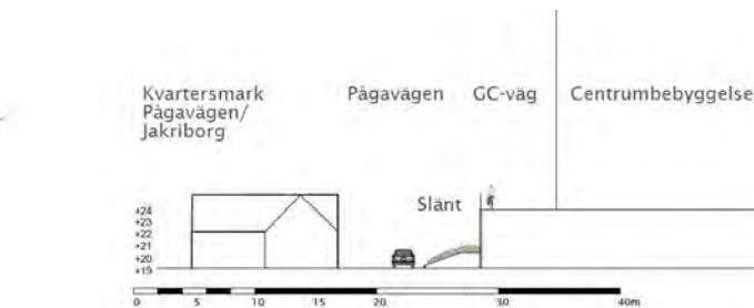
Figur 6. Sektion B-B. Småhusbebyggelsen i västra delen av planområdet, Arkitektlaget.
