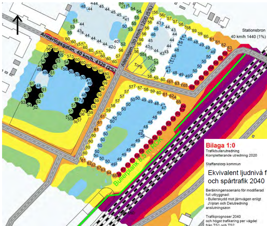
Figur 19. Utdrag ur "(PM Bullerutredning Västerstad, Sweco 2020-12-16 - delutredning 2". Denna bullerutredning kompletterar den som visas på föregående sida och utreder bullersituationen för planområdets östra del. Ljudspridningskartorna visar tydligt att 60 dBA ej överskrids inne på gårdarna. Förutsatt att lägenheter exempelvis utförs genomgående så klarar bebyggelsen gällande riktlinj för buller.
