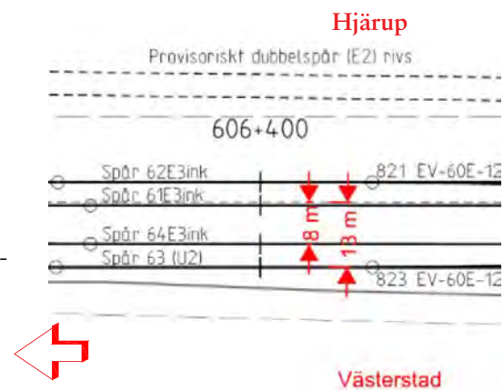
Figur 15. Utdrag från risikutredningen. Bilden visar placering av provisoriska spår (fram till september 2022) samt spårnummer på framtida permanenta 4 spår genom Hjärup.
